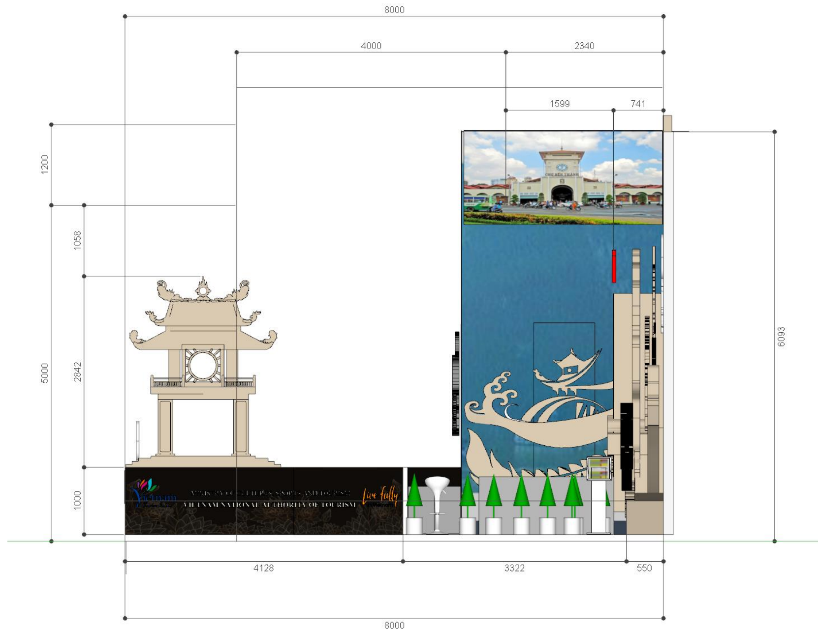
Sơ đồ mặt đứng gian hàng
