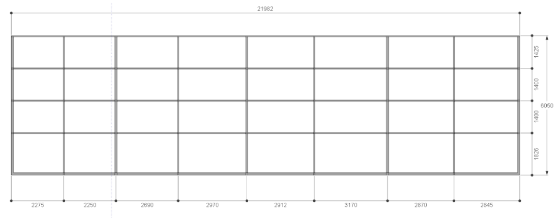
Hệ thống khung xương sắt
