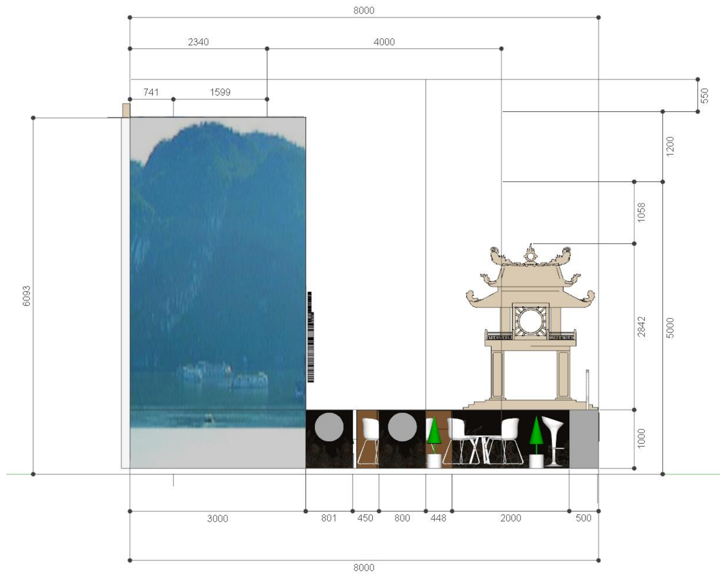
Sơ đồ mặt đứng gian hàng
